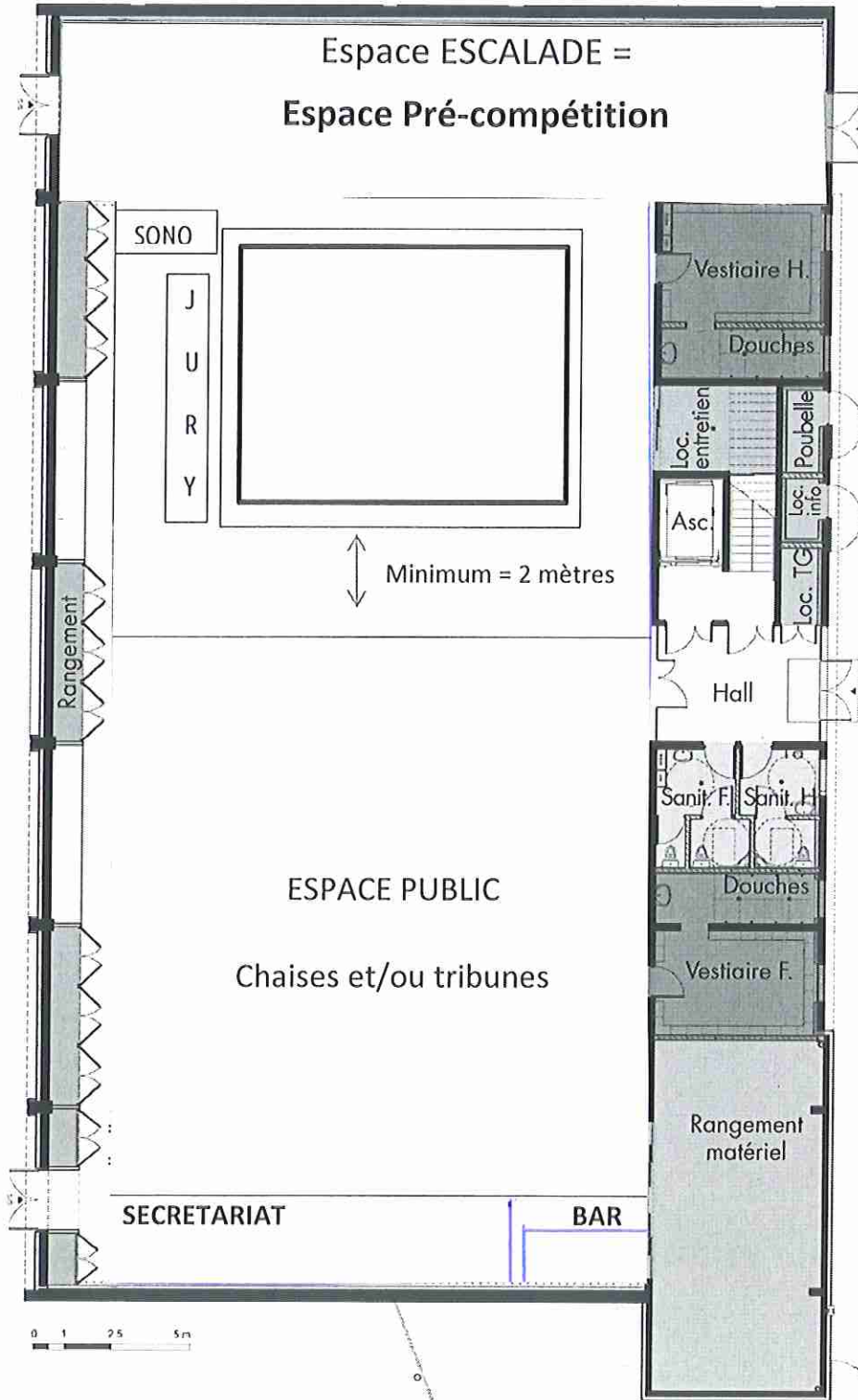
Plan du niveau 0
