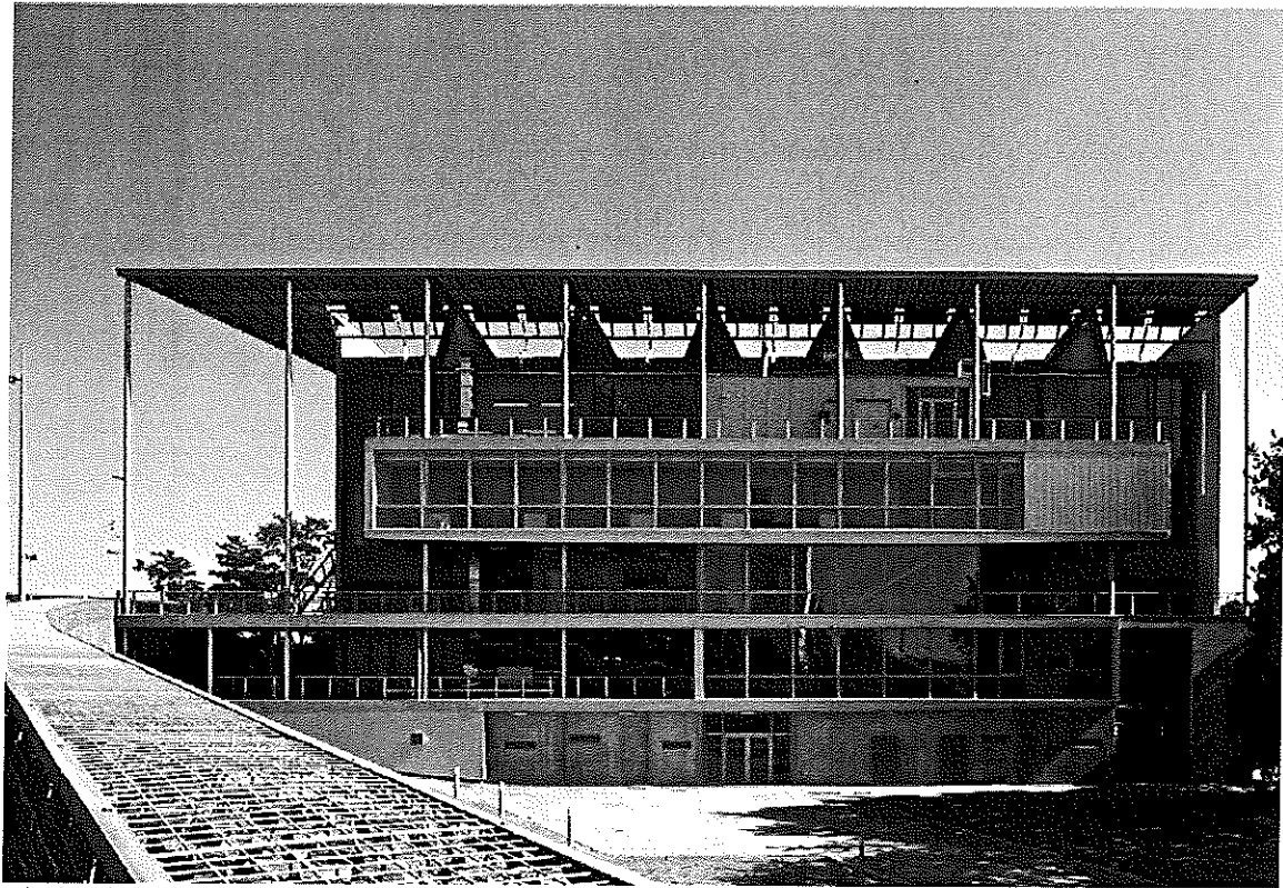
La façade Nord et ses coursives, à l'Ouest le mur en gabions
